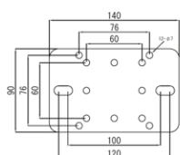
【スピーカーベース】
