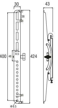
【モニター側】 【側面】
