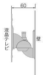
【側面】
