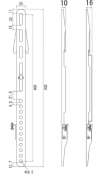
【モニター側金具】 【側面図】
