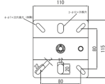
【天井ベース】
