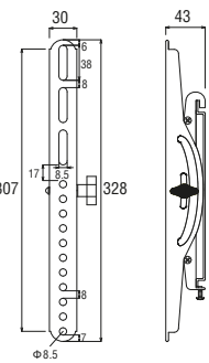
【モニター側】 【側面】
