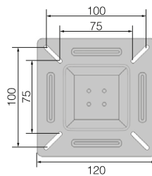
【テレビ側】
