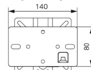
【天井ベース】
