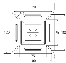
[テレビモニター取付面]
