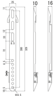
【モニター側金具】 【側面図】
